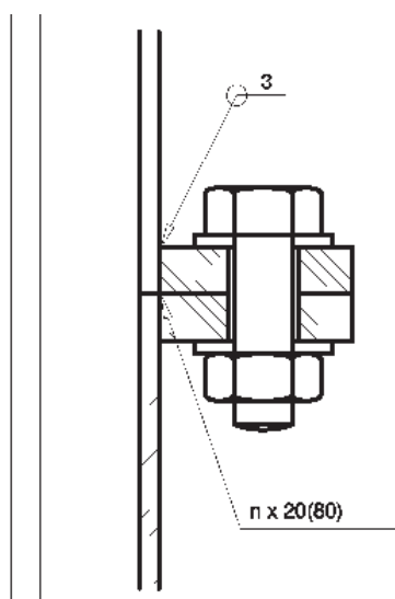
Fig. 2. Flangesamling med svejste flanger
