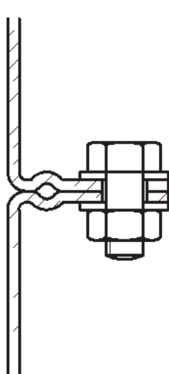
Fig. 1. Flangesamling med bertlede flanger
